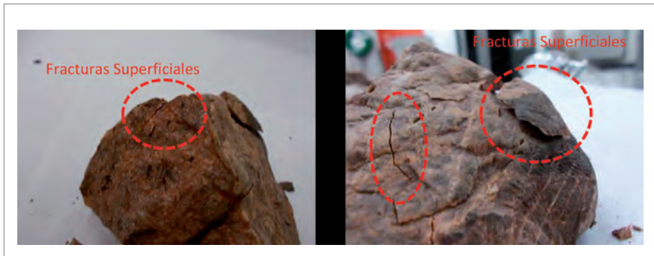
Figura 28 - Roca expuesta a 100 \text{ kW/m}^2 por 30 min de manera homogénea (22 de julio, 2015).
