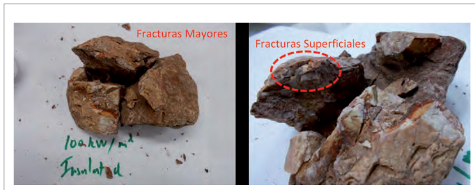
Figura 28 – Roca expuesta a 100 \text{ kW/m}^2 por 30 min en una cara con la otra cara aislada térmicamente (22 de julio, 2015).
